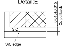
Detail:E
